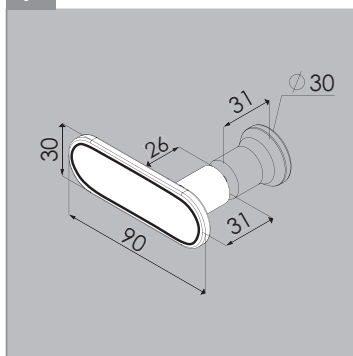
F UCHWYT
