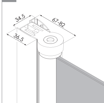
A PROFIL PRZYŚCIENNY
