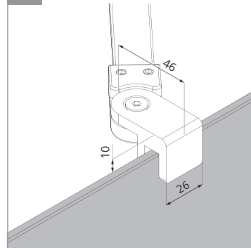
D WSPORNIK
