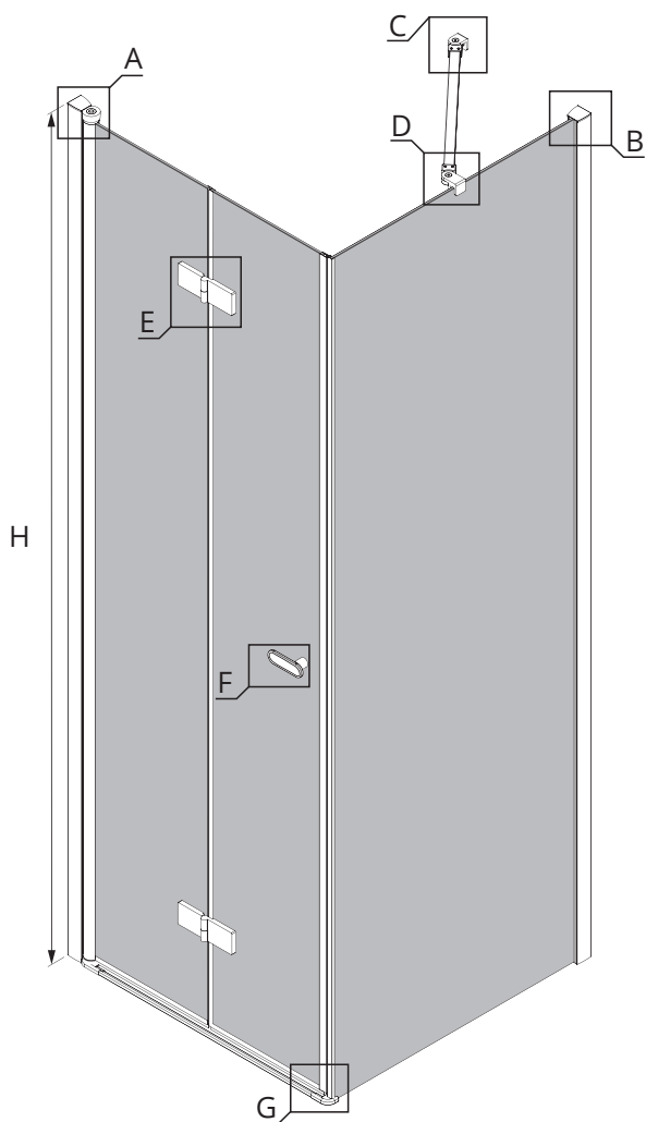
A PROFIL PRZYŚCIENNY
