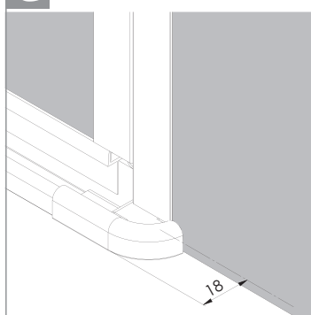
G ZAKOŃCZENIE PROGU
