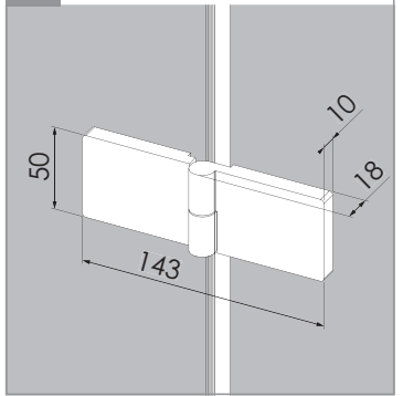
G UCHWYT
