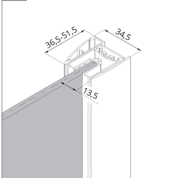
C UCHWYT
