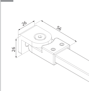
D WSPORNIK
